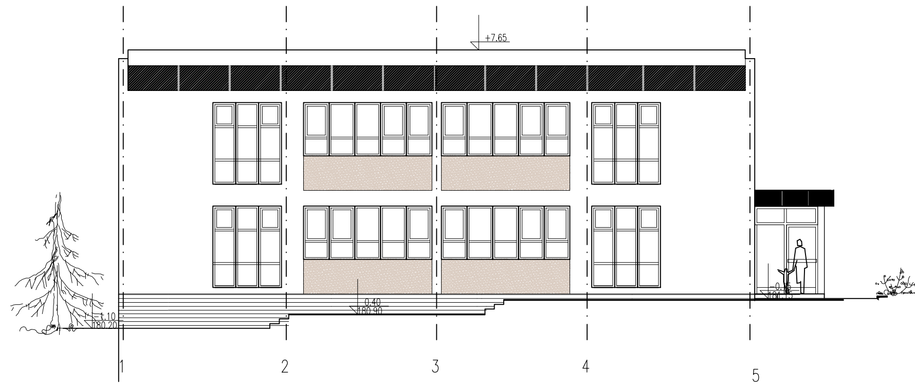
ЈУГОИСТОЧНА ФАСАДА
