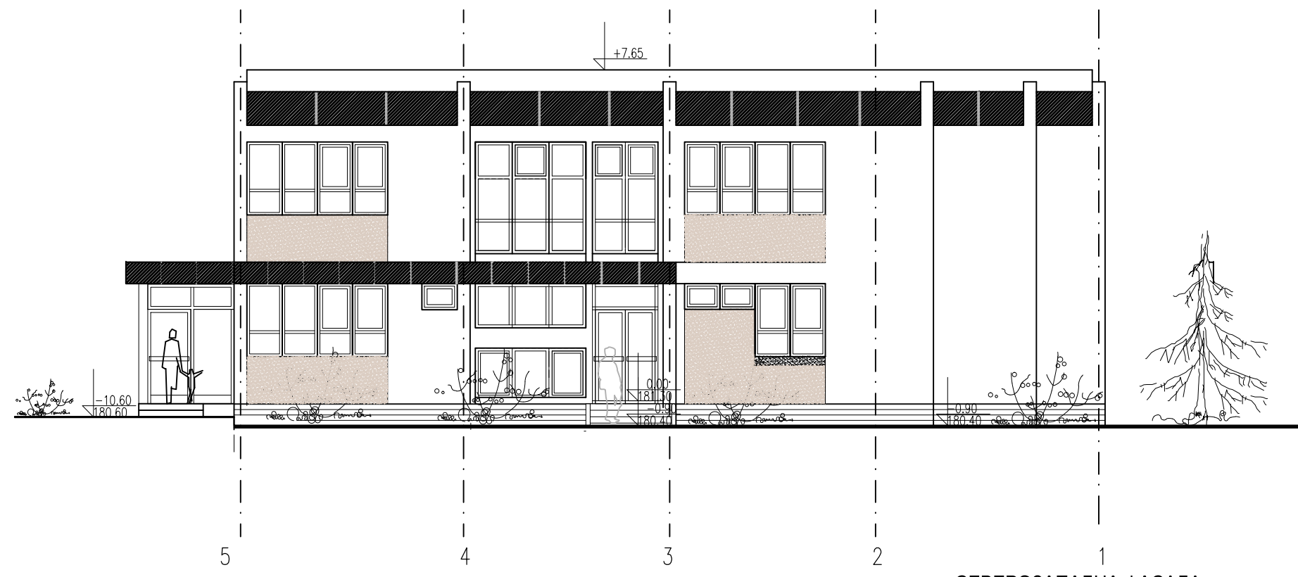
СЕВЕРОЗАПАДНА ФАСАДА
